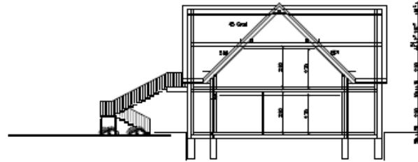
Schnitt B.-B.
