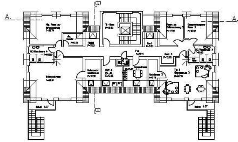
Dachgeschoss
