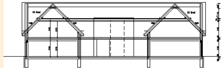
Schnitt A.-A.
